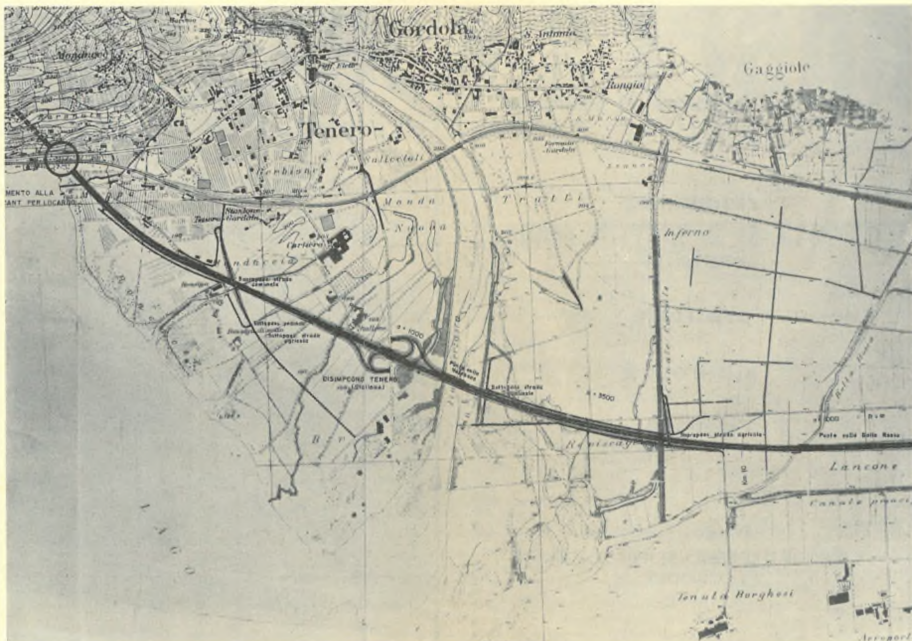
Progetto della nuova strada cantonale
