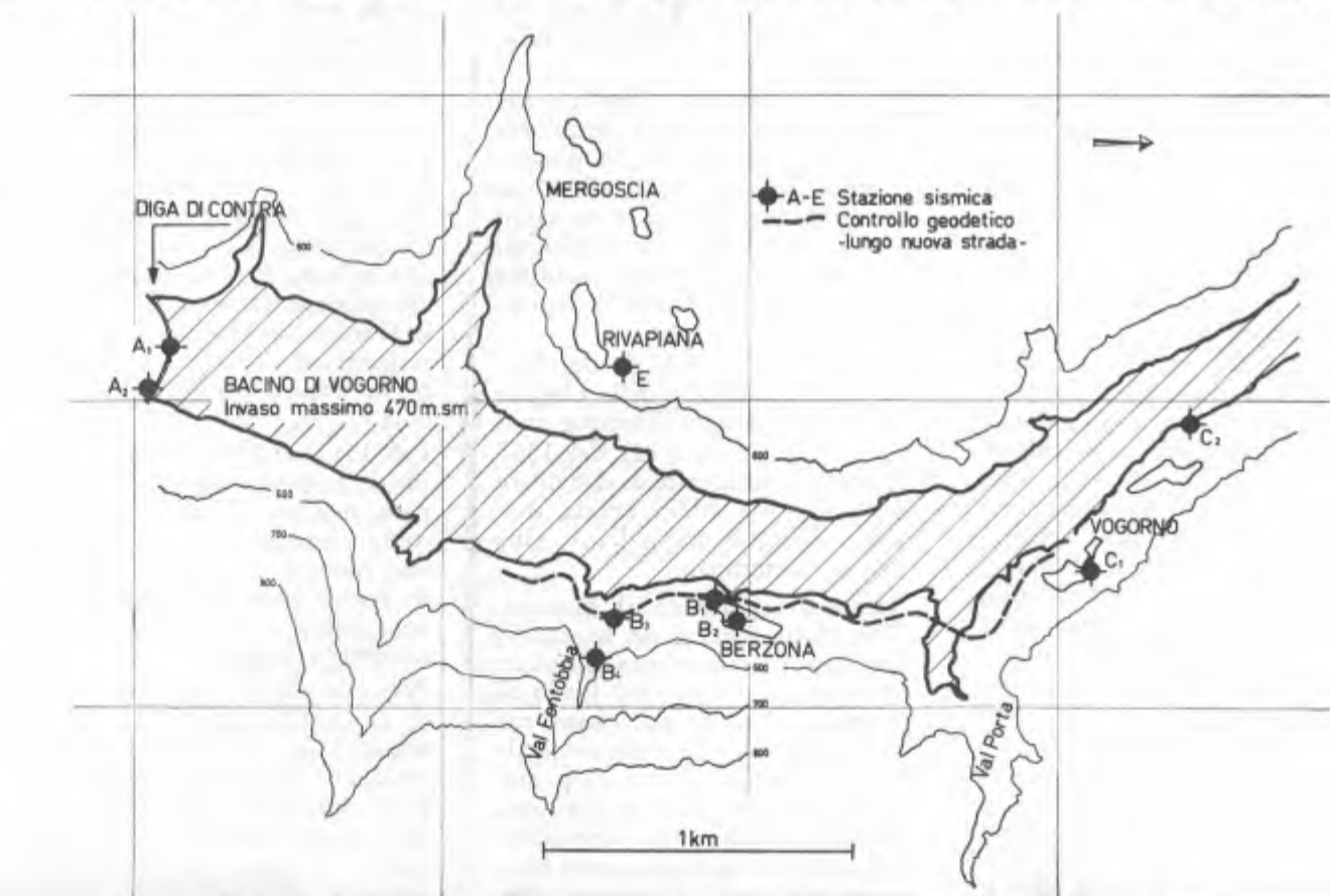
Planimetria del lago di Vogorno. Ubicazione dei sismografi per il controllo.
